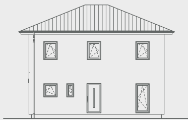
Ansicht Eingang
